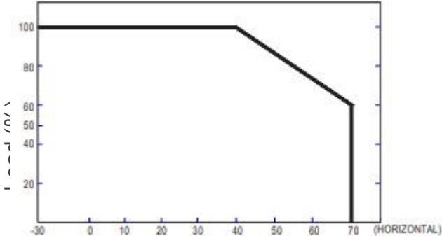
Environment temperature(°C)
