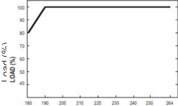
Input voltage(VAC)
