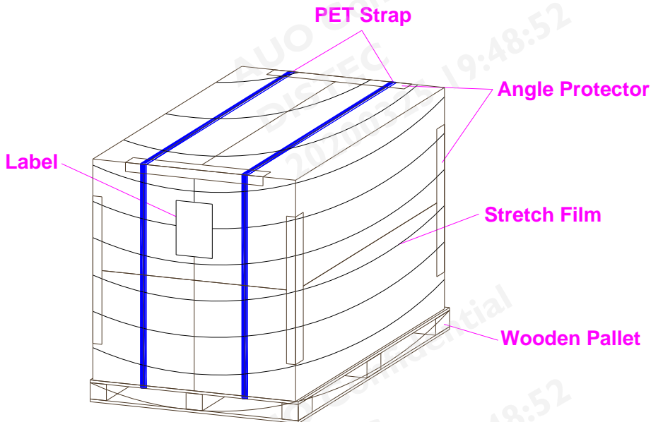
單棧 pallet 打棧示意圖
